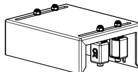
art. 463 Piastra di guida 4 olive schermate
