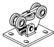
art. 395-P Carrello di guida
